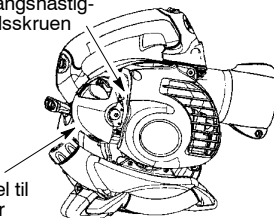
Tomgangshastighedsskruen
