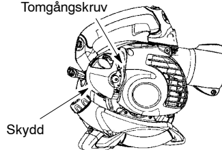
Tomgångsskruv
